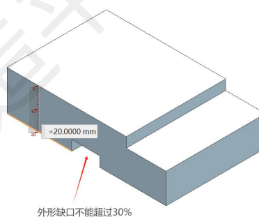
标准厚度双面特征
