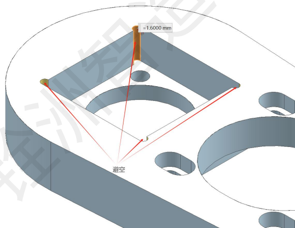
内直角避空设计
