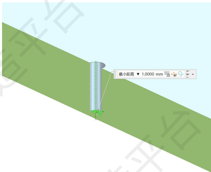
攻牙孔底需预留足够壁厚
